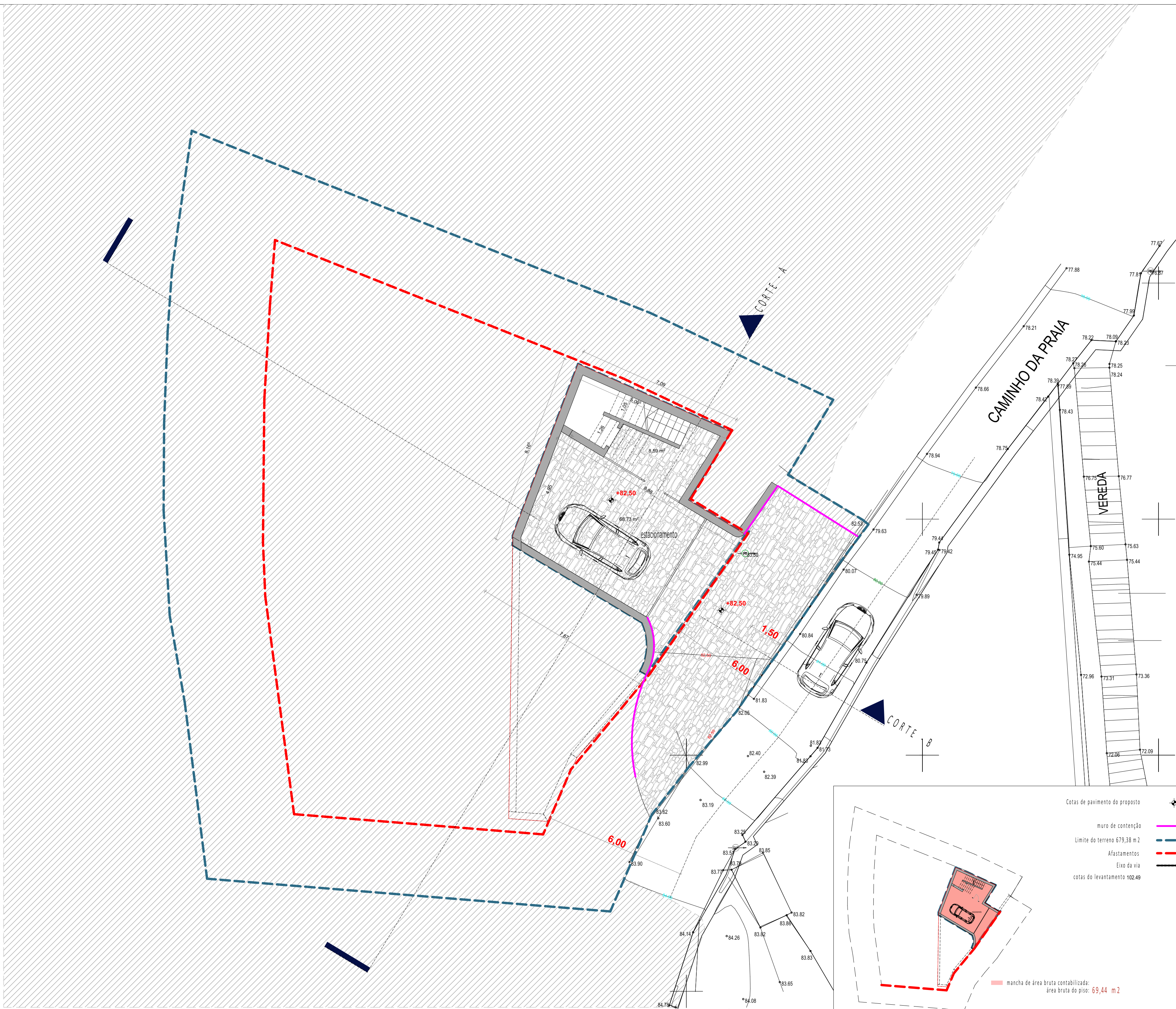
PLANTA DA GARAGEM
